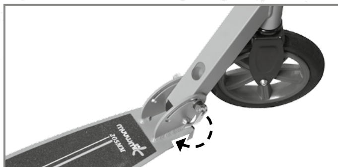
Déplier le guidon.
